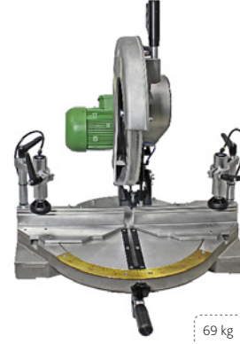
HA 1014 Portatif Pnö. Sıklı Tek Kafa Kesim Makinası
